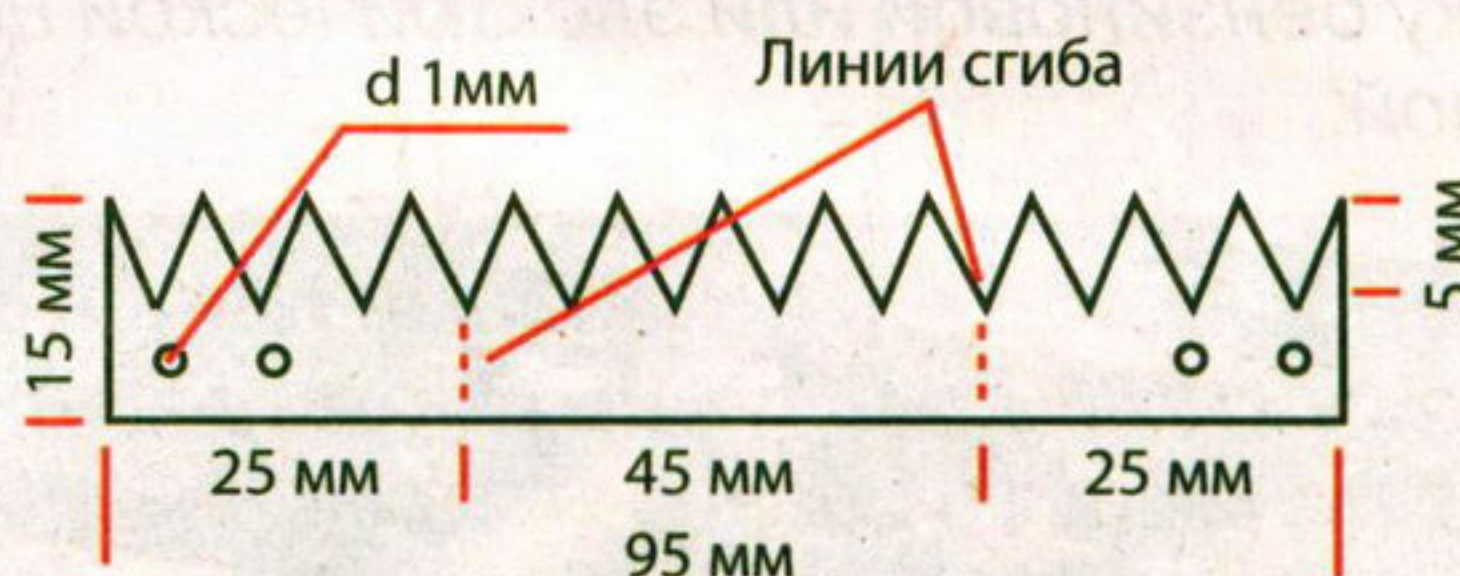
Рис. 2 Мышеловка в сборе
