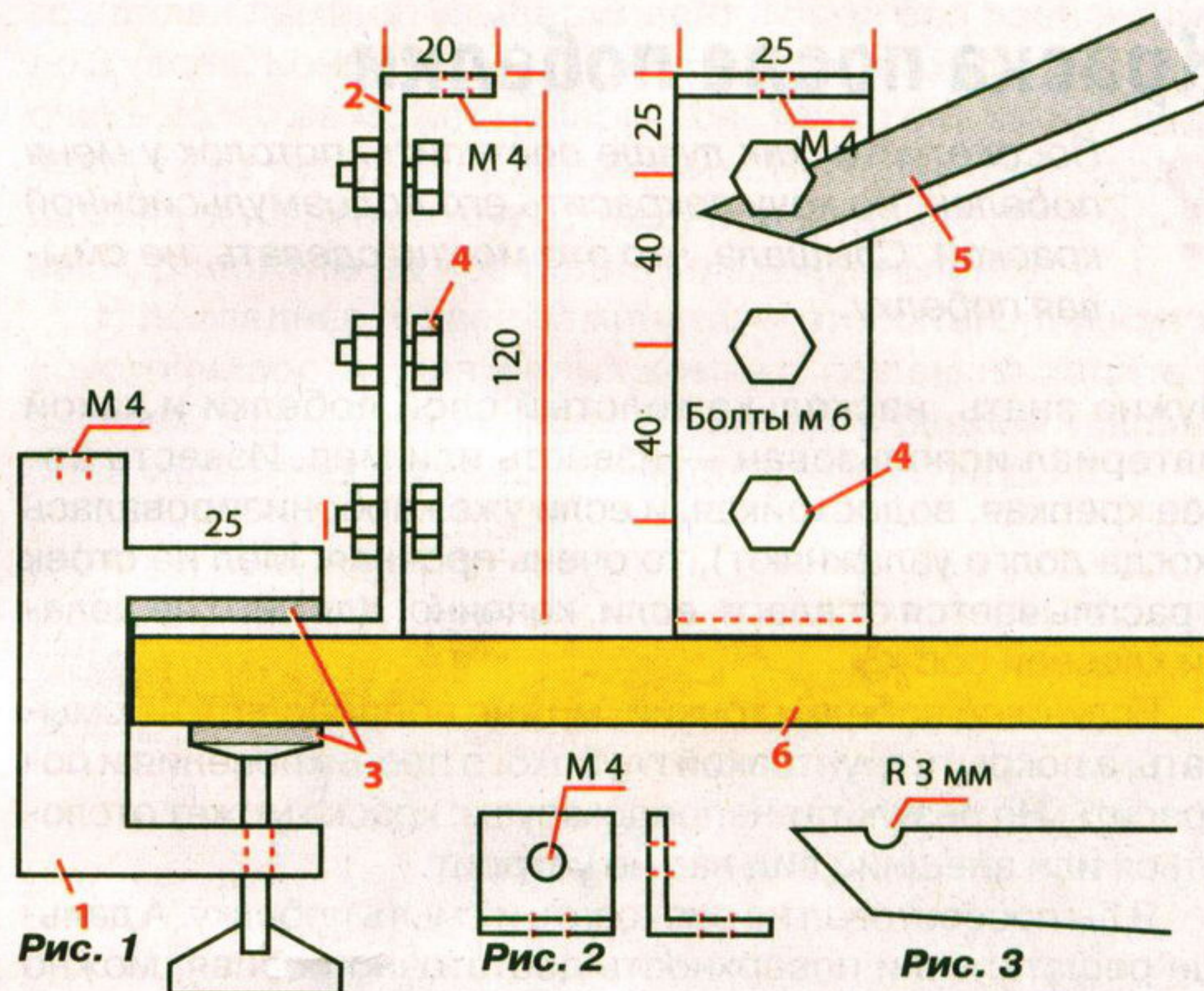
Чертеж ножа
