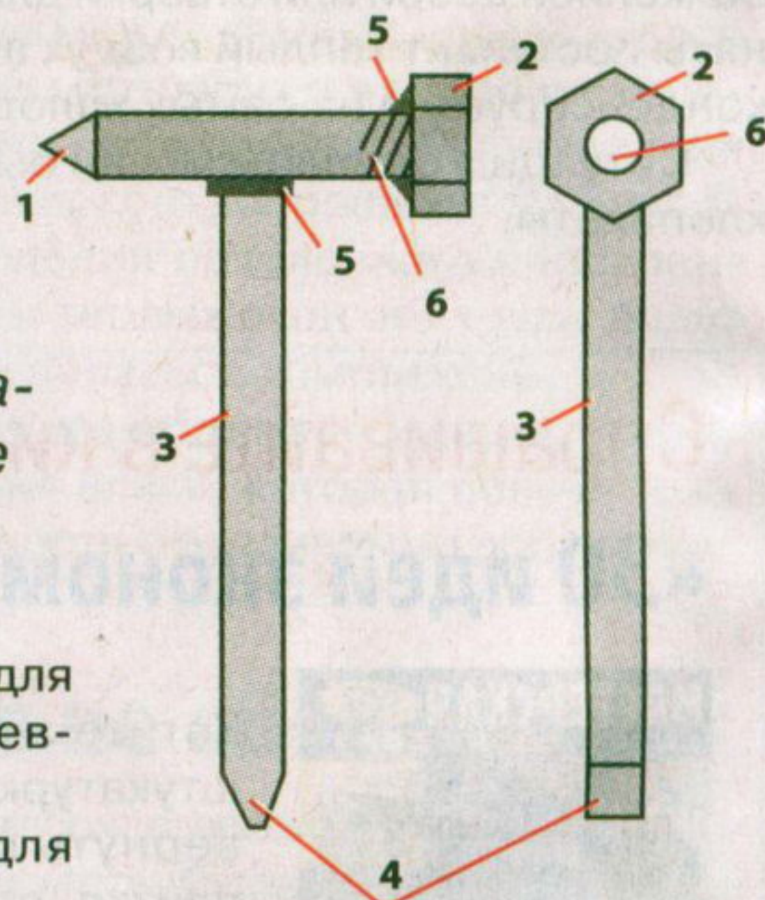
На рис. 1 — острый конец для кернения, 2 — гайка-молоточек, 3 — стальной палец, 4 — заостренная отвертка, 5 — место сварки, 6 — шпилька с резьбой
